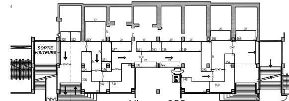
Niveau 300
